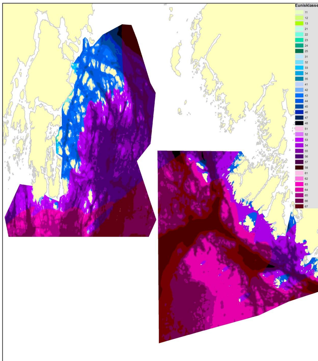
Figur 32. Oversikt over utbredelse av EUNIS-klasser i utredningsområdet for Ormø-Færder og i Ytre Hvaler nasjonalpark. Symbolforklaringen viser hvilke fargekode som representerer de ulike klassene. Det første tallet viser bølgeeksponeringsklassen, og det andre tallet dybdeklassen som fargen representerer. Dess mørkere farge dess dypere områder. Det er angitt en fargetype per eksponeringsklasse. Målestokk 1:200 000.
