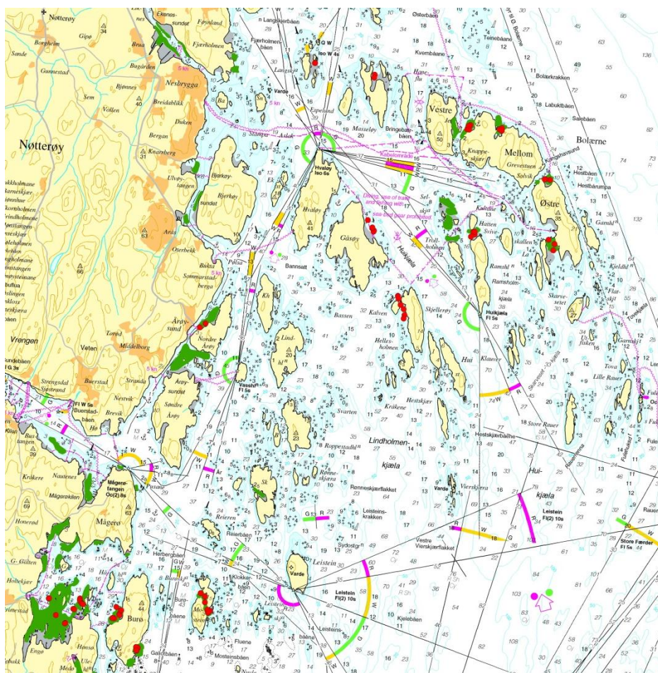
Figur 10. Funn av ålegras (røde punkter) i den nordlige delen av utredningsområdet. Røde punkter uten grønn bakgrunn er ikke inkludert i Naturbasen. Grønne felter er tidligere kartlagte forekomster. Målestokk 1:50 000. (Bakgrunnskartet er fra hovedkartserien til Sjøkartverket.)
