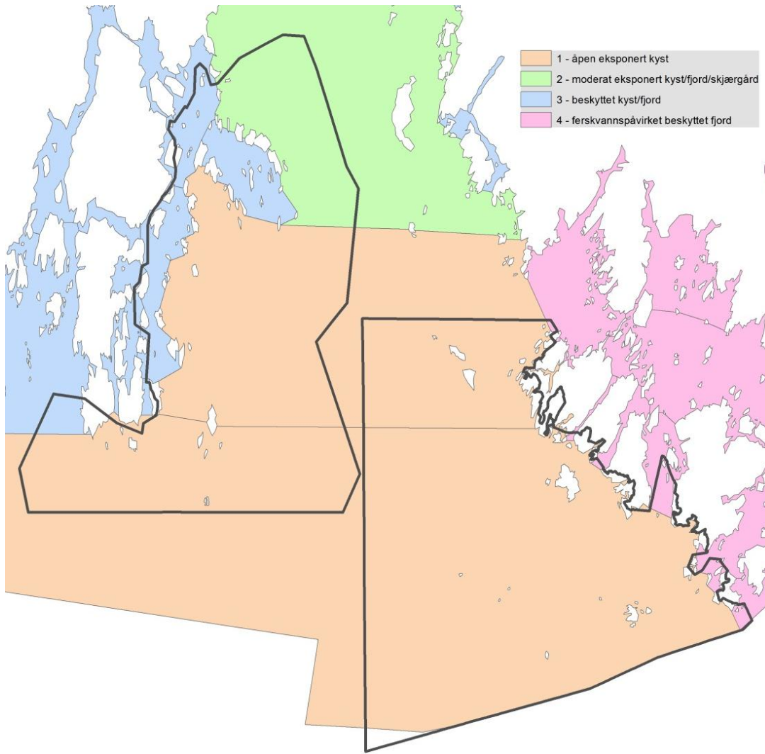
Figur 31. Oversikt over hvilke vanntyper som finnes ved Ormø-Færder og ved Ytre Hvaler i henhold til Vanndirektivet. Målestokk 1:120 000.
