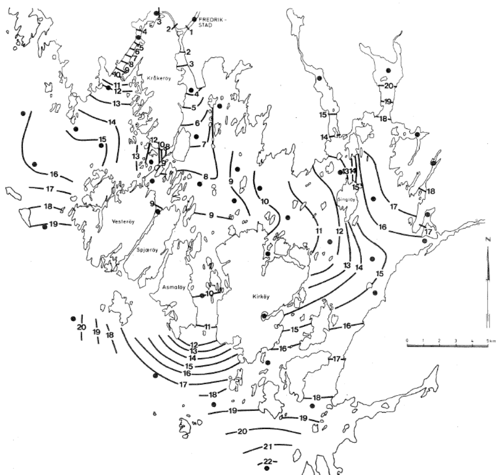
Figur 35. Overflatesaltholdighet (promille, 0,5 m dyp) i Hvalerområdet og Singlefjorden. Middelverdier av fem tokt i 1980 – april, juni, juli, august, september. (Fra Magnusson og Skei 1984).
