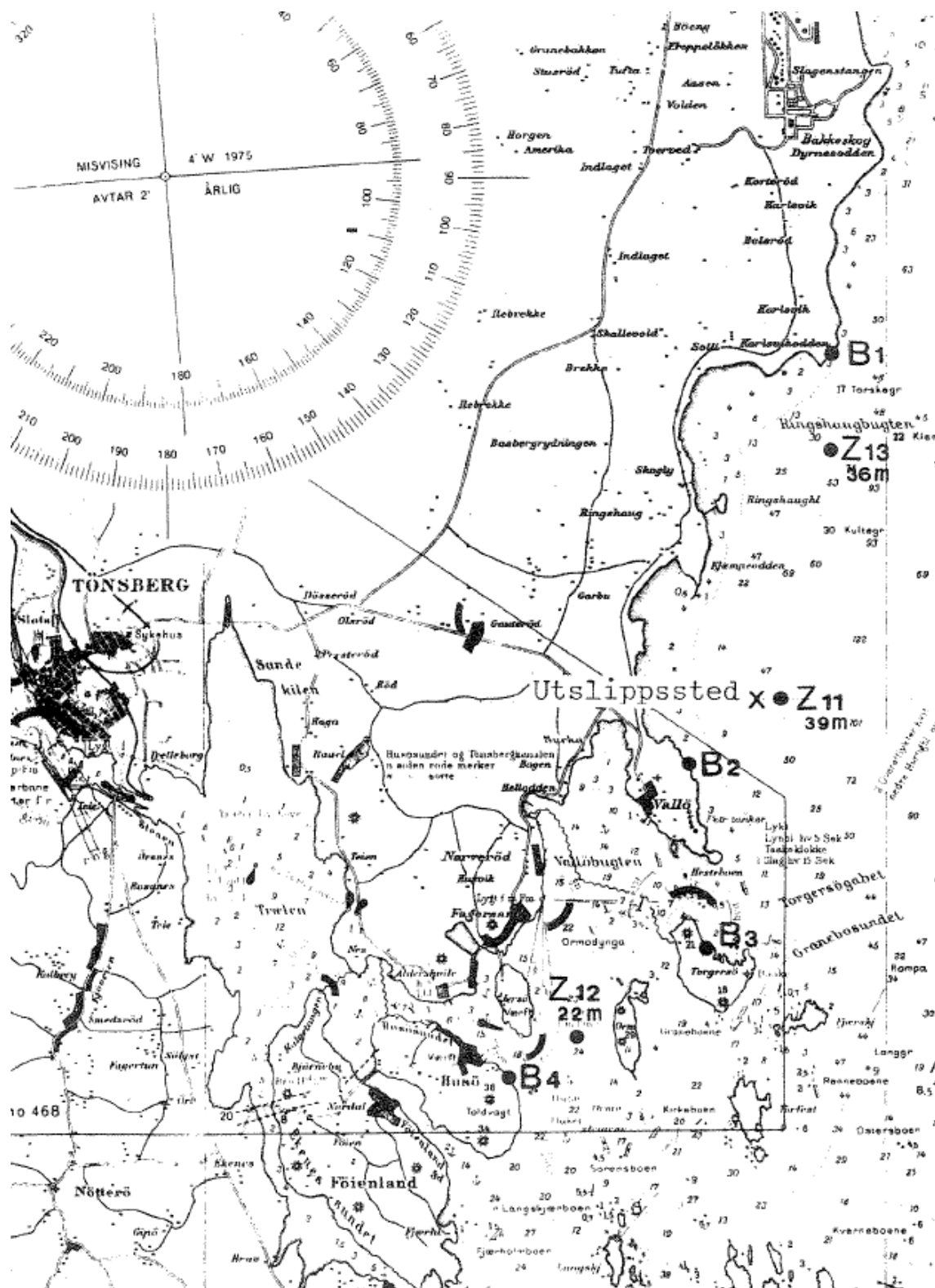
Figur 37. Oversikt over gruntvannsstasjoner og bløtbunnstasjoner som det ble gjort biologiske undersøkelser av i 1978 tilknyttet en resipientundersøkelse utført av NIVA innen utredningsområdet (Kvalvågnæs og Rygg, 1979).
