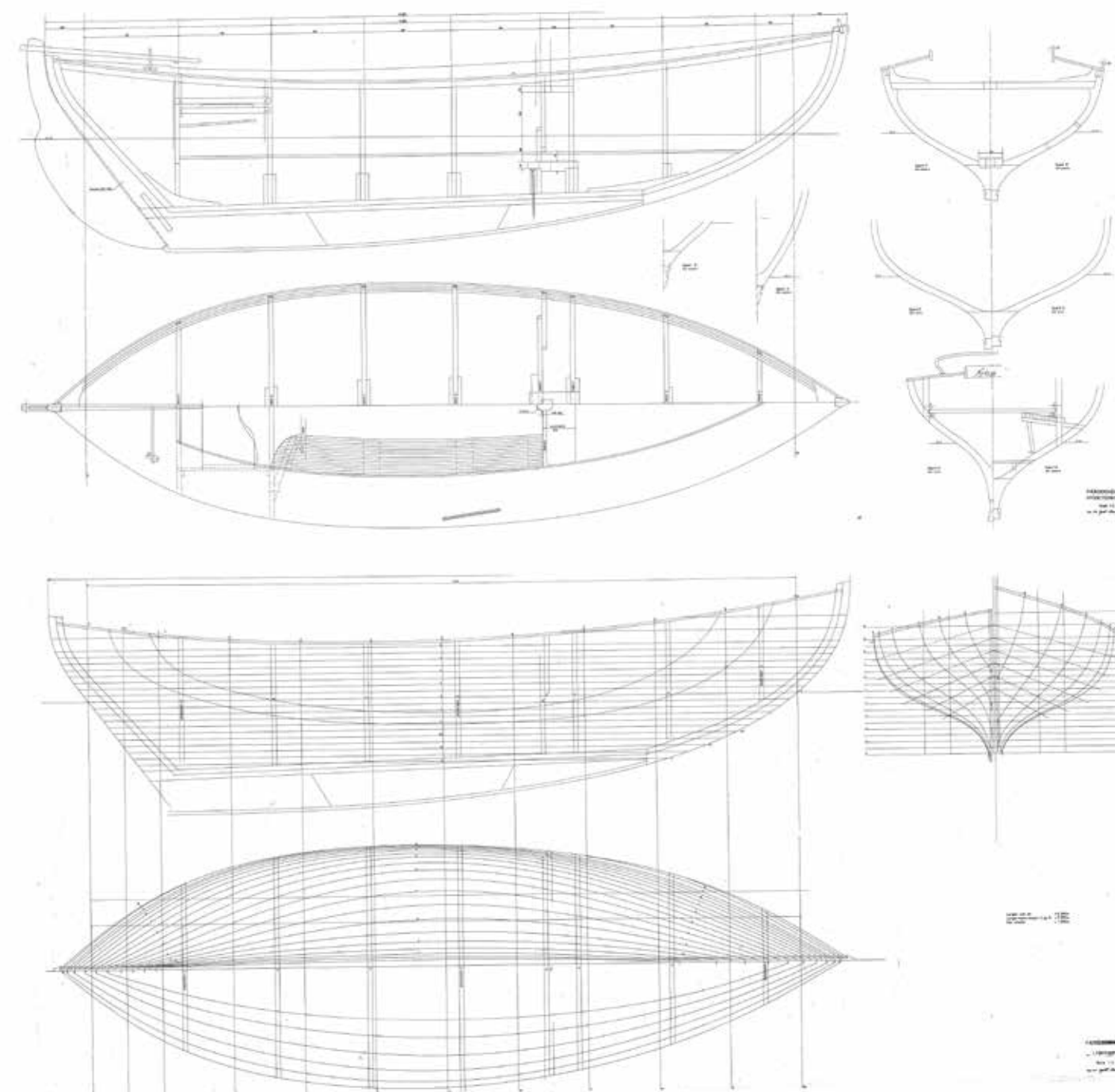
Byggetegninger / Boat plans
